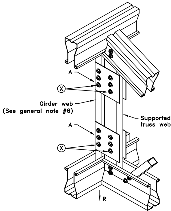
2 Clip Connection**
